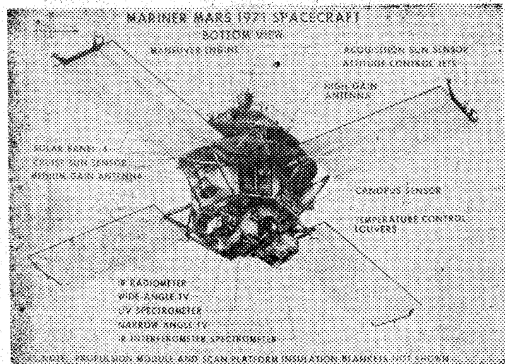
Así es exactamente el "Mariner 9"
