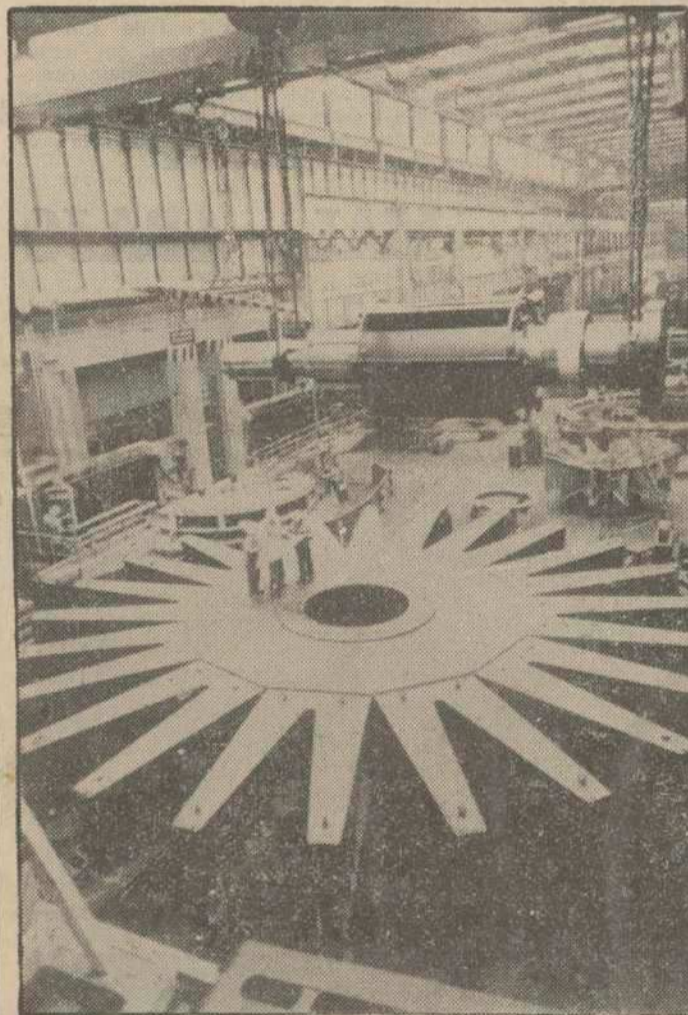
La fotografía nos muestra uno de los momentos del montaje de uno de los dos generadores más grandes que se han construido hasta ahora en la fábrica de Siemens en Berlín. Están destinados a una central eléctrica de Argentina y tienen, cada uno, una potencia de 240.000 kilowatts. El diámetro del rotor de tan monumental generador es de 16 metros. — (Foto FIEL)
