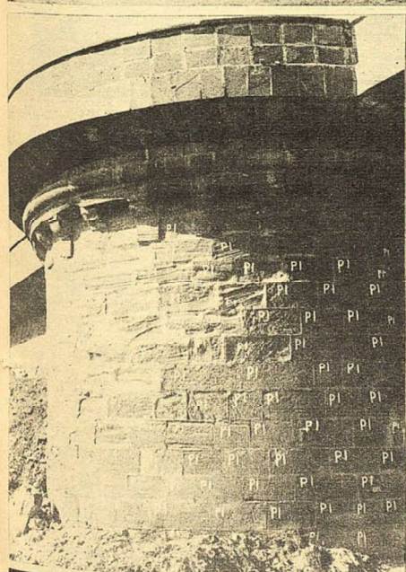
Los primeros trabajos para el desmonte y traslado del bicentenario puente de Molins de Rei sobre el Llobregat, comenzaron por la numeración, uno a uno, de los bloques de las pilastras del viaducto, operación que luego ha de facilitar la reconstrucción de la obra, en el lugar en que se acordó situarlo de nuevo y del que todavía no se tiene noticia concreta. Se trabaja a buen ritmo al objetivo de cumplir el plazo fijado para el 30 de abril próximo, en que ha de iniciarse la obra del nuevo puente de seis carriles de circulación. Otro puente, de cuatro carriles, está casi terminado en su parte más importante. En este caso se cumplirá también el plazo marcado de cincuenta días para poder cruzar de nuevo el Llobregat en aquella zona. — (Fotos Postluis)
