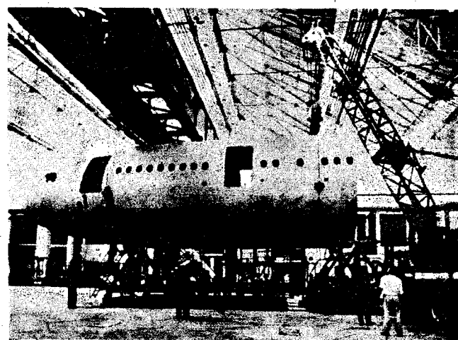
Colocación en el armazón de ensambladura del tramo delantero del fuselaje del "Airbus" A 300 B.
