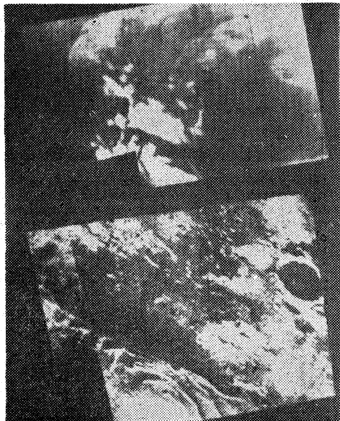
Polo Sur de Marte La foto superior muestra el polo Sur del planeta Marte, cubierto parcialmente por una nube de polvo, tal como ha sido captado el domingo por el "Mariner 9". La foto inferior muestra la misma sección del planeta captada por la cámara del "Mariner 7" en 1969. La foto superior ha sido captada por el Jet Propulsion Laboratory, de Pasadena (California). (Foto Europa Press.)
